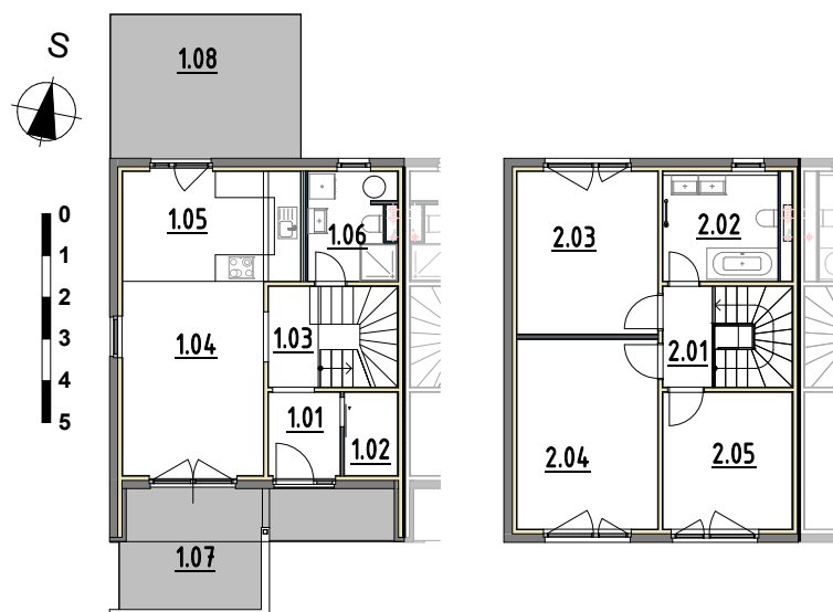
PŮDORYS 1.NP
