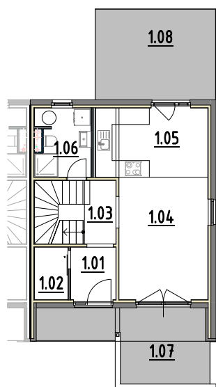
PŮDORYS 1.NP
